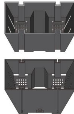
<내·외부 케이스 뒷면 에어홀 구조>
