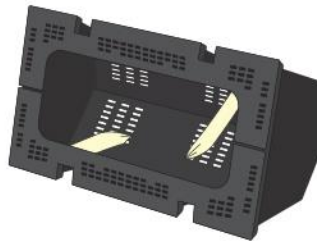
양털 심지를 장착한 내부케이스 Biowall Incase Pot
